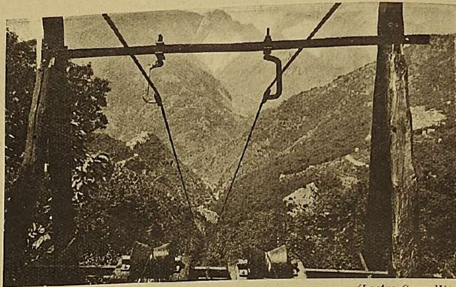
(Lastre Cappelli). Una teleferica alle cave dei marmi (fot. Pampaloni).
