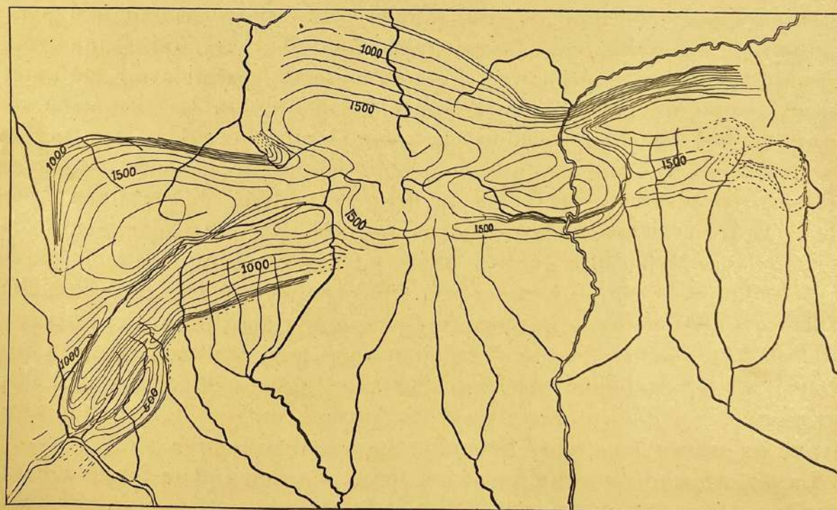
FIG. 55-56. — Extension des niveaux d'érosion et déformation de la plate-forme Riu Ses. 1, plate-forme pliocène ou de Govornitza; 2, plate-forme Riu Ses; 3, régions où l'érosion a fait disparaître la plate-forme Boresco sans que le modelé ait été poussé jusqu'à la maturité pendant le stade Riu Ses; 4, plate-forme Boresco; 5, témoins anciens d'érosion au-dessus de la plate-forme Boresco.
