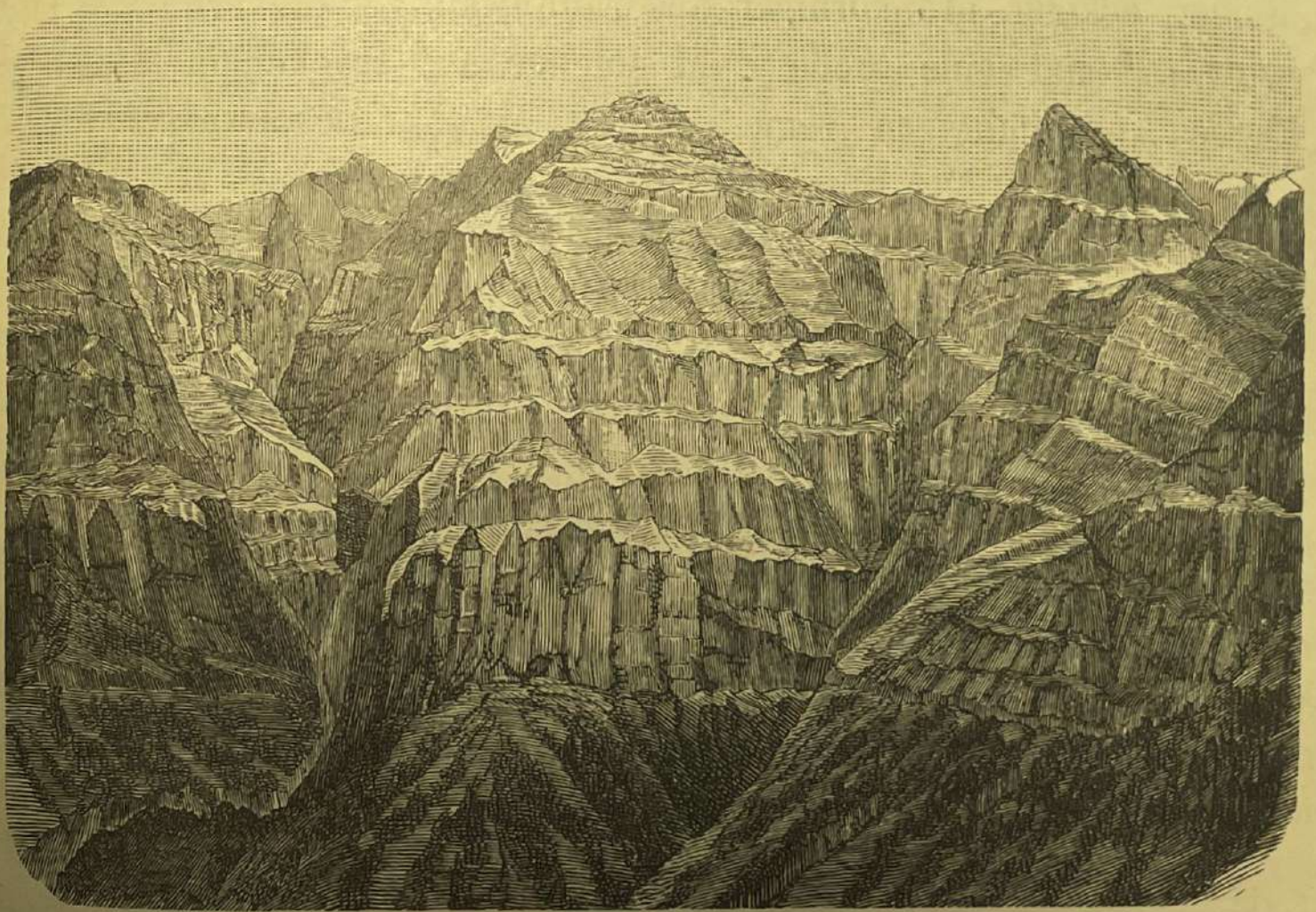
Fig. 116. Verwitterungsterrassen im Glärnisch-Gebirge nach BALTZER.
