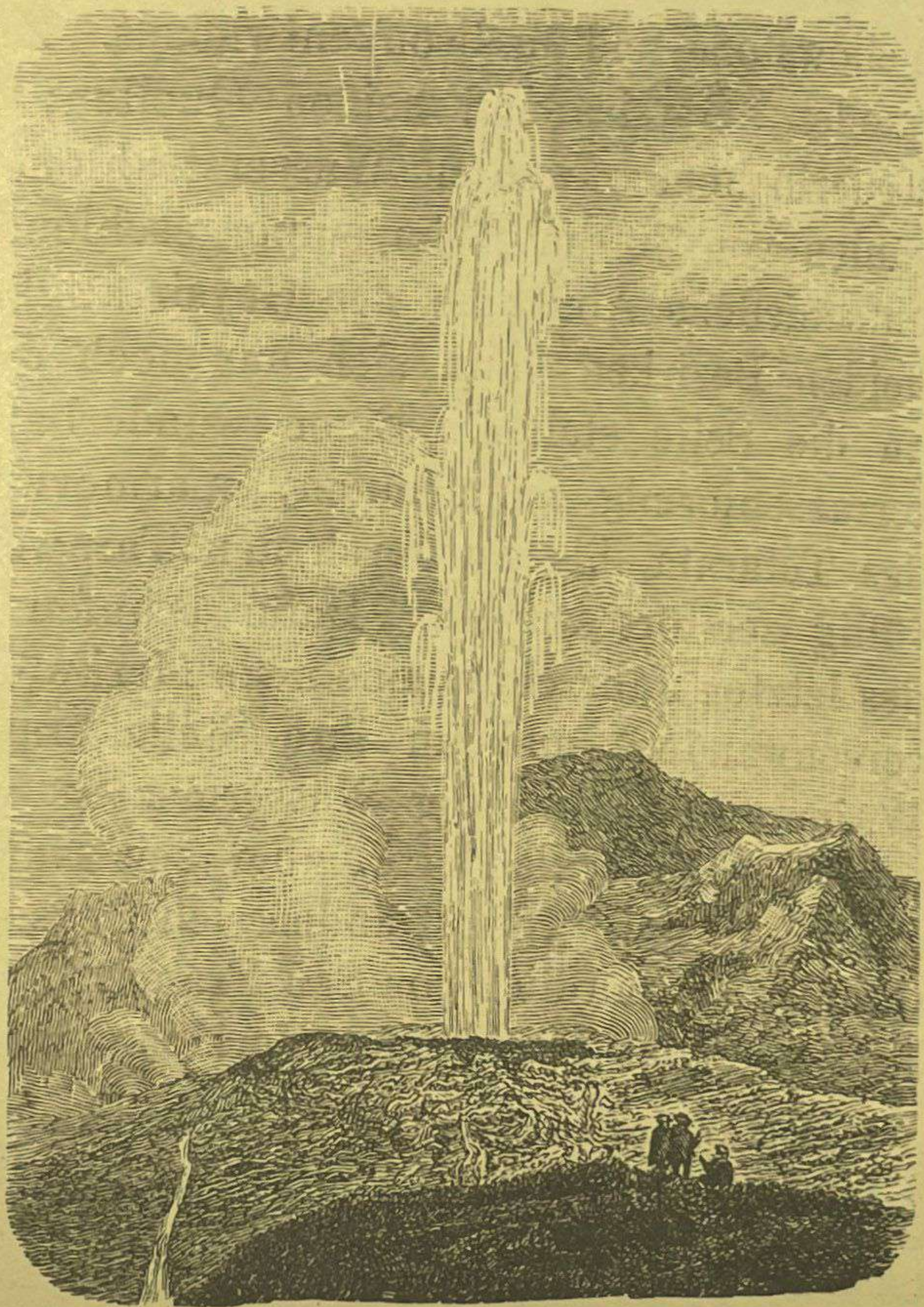
Fig. 125. Der Große Geysir nach K. FUCHS.
