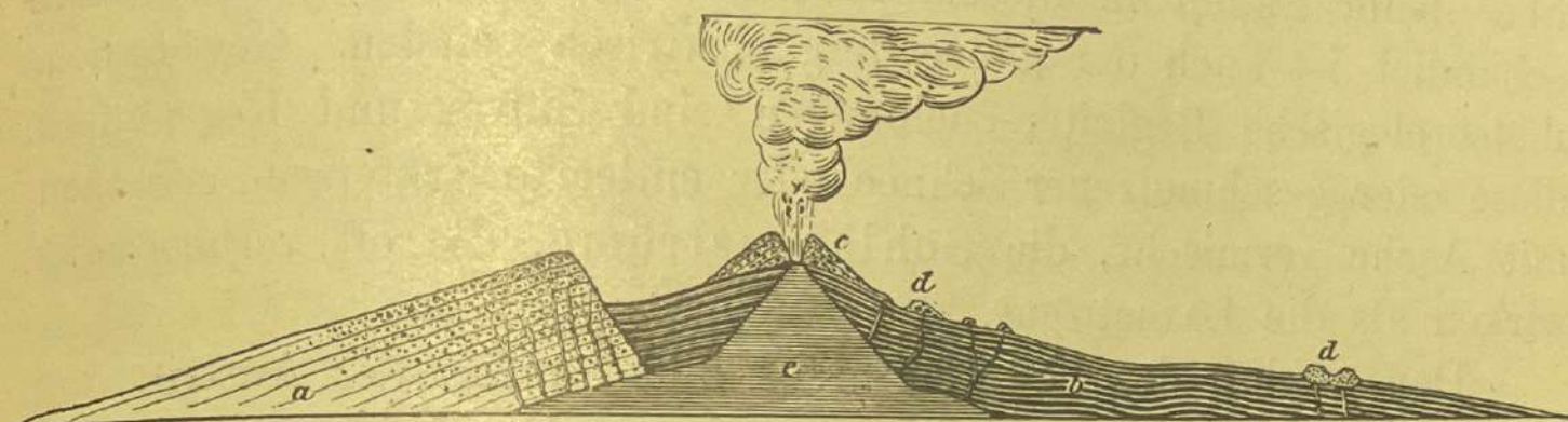
Fig. 97. Idealer Durchschnitt des Vesuvs nach von HOCHSTETTER.
